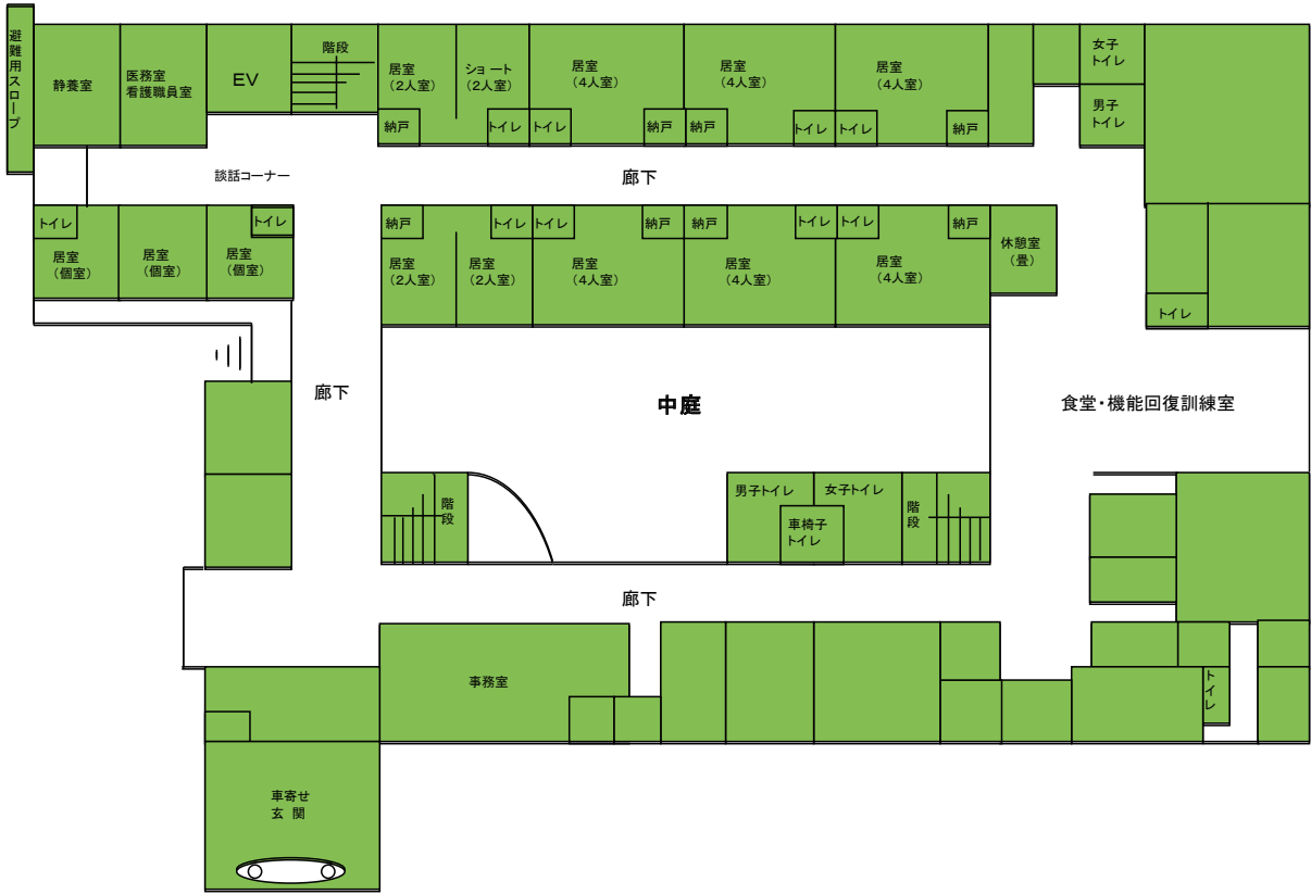
(愛灯園 二階 平面図)
